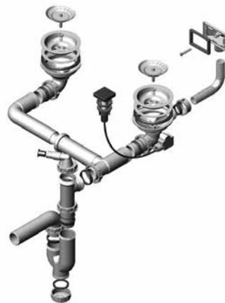
Syfon podwójny POP-UP 2XQM 114 - PP - 114 POP - UP
