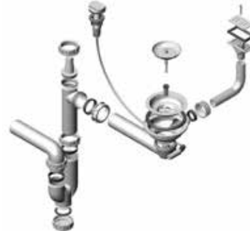
Syfon pojedynczy POP-UP 1XSP 114-HP POP-UP-N ECO
