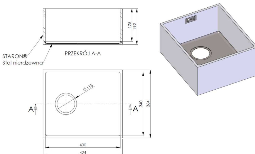
Rys. 2 Komora duża zlewozmywaka
