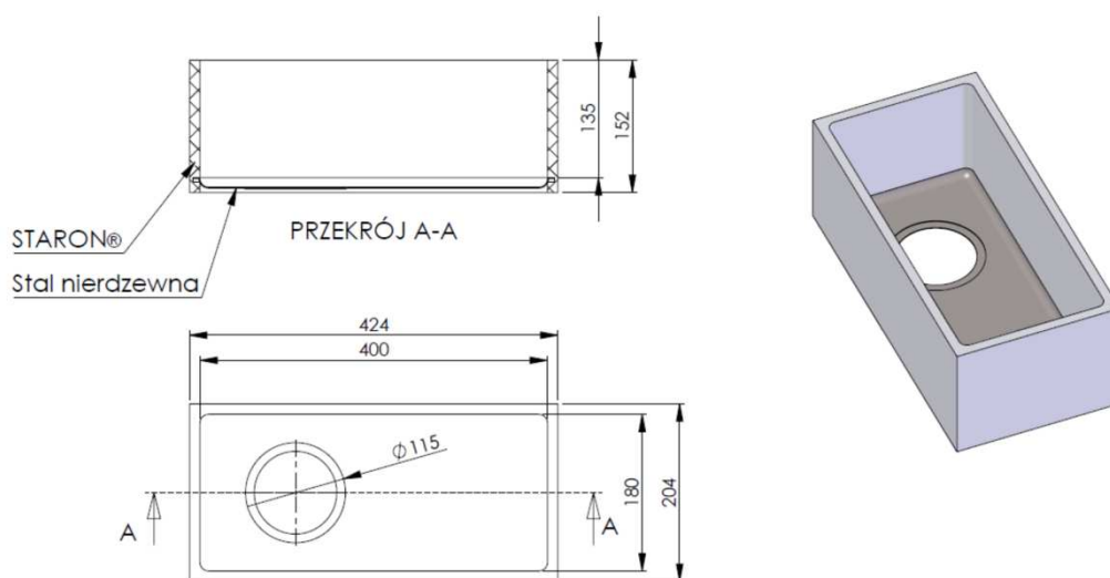
Rys. 1 Komora mała zlewozmywaka
